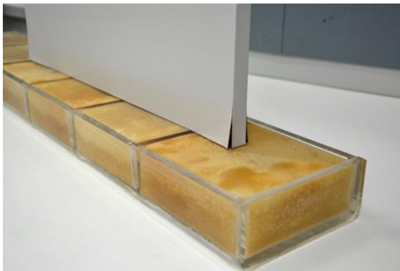
Figura 46. Prova di resistenza dei bordi all'acqua
